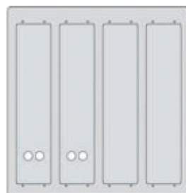
Art. 1E34 pro 4 panely výška 3 moduly. Rozměr čelní 424x412x74 mm Rozměr zadní: 420x410 mm (ŠxV)
