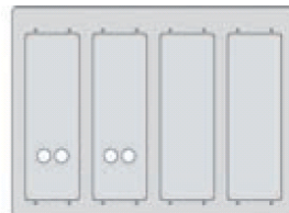
Art. 1E24 pro 4 panely výška 2 moduly. Rozměr čelní 424x297x74 mm Rozměr zadní: 420x295 mm (ŠxV)
