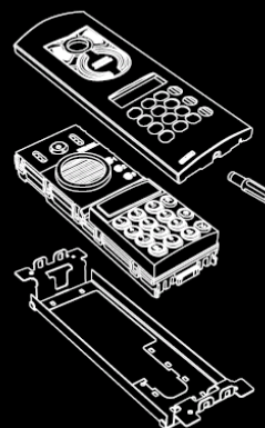
Instalace na povrch s rámečkem proti dešti.
