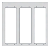
Art. 1P23 pro 3 panely výška 2 moduly. Rozměr čelní 324x297x39,5 mm Rozměr zadní: 320x295 mm (ŠxV)
