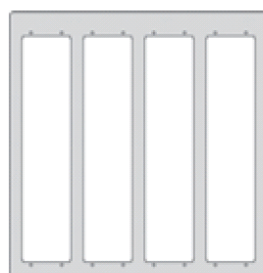
Art. 1P34 pro 4 panely výška 3 moduly. Rozměr čelní 424x412x39,5 mm Rozměr zadní: 420x410 mm (ŠxV)
