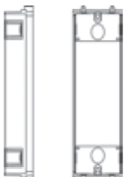
Art. 9092 nebo 9192 Rozměry: 88x248x50 mm
