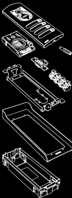
Instalace panelu zapuštěného do zdi s rámečkem proti dešti.
