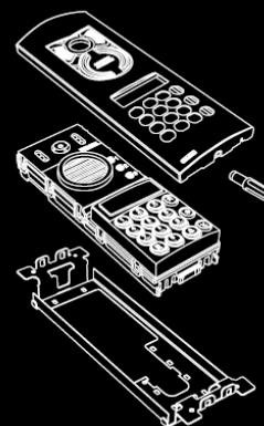
Do panelu audio nebo video s alfanumerickou klávesnicí a displejem, pro zařízení Due Fili nebo DigiBus, je potřeba vložit: pouze alfanumerickou jednotku elektroniky audio nebo video.
