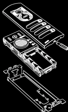
Do panelu audio nebo video s tlačítky, pro zařízení Due Fili nebo DigiBus, je potřeba vložit: pouze jednotku elektroniky audio nebo video s tlačítky.
