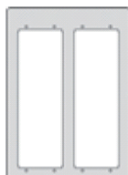
Art. 1P22 pro 2 panely výška 2 moduly. Rozměr čelní 224x297x39,5 mm Rozměr zadní: 220x295 mm (ŠxV)
