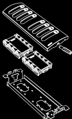
Do přídatného panelu s tlačítky, pro zařízení Due Fili nebo DigiBus, je potřeba vložit: pouze přídatné moduly s tlačítky art. 12TS.
