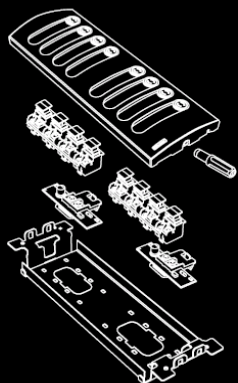
Do přídatného panelu s tlačítky, pro zařízení s výzvou Sound system nebo ac, je potřeba vložit: LED osvětlení jmenovek art. R260 jedno pro 4 tlačítka a tlačítka art. R200 nebo R200/50.
