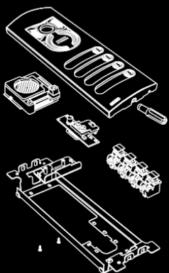
Do panelu audio nebo video s tlačítky, pro zařízení s výzvou Sound system nebo ac, je potřeba vložit: hovorovou jednotku nebo kameru s hovorovou jednotkou, LED osvětlení jmenovek art. R260 jedno pro 4 tlačítka a tlačítka art. R200 nebo R200/50.
